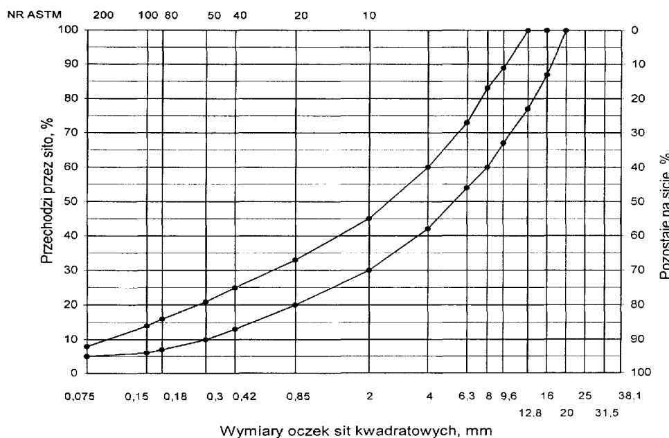
Rys. 2. Krzywe graniczne uziarnienia mieszanki mineralnej BA od 0 do 16 mm do warstwy wiążącej, wyrównawczej nawierzchni drogi o obciążeniu ruchem od KR3 do KR6
